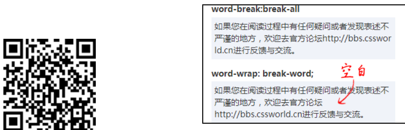
图 8-36 word-break:break-all 和 word-wrap:break-word 效果区别
