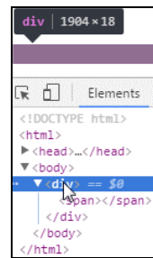
图 3-29 高度不为 0 证明幽灵空白节点的存在（截自 Chrome 浏览器）
